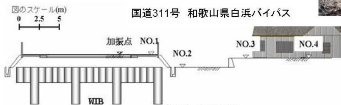
図-2 断面図
