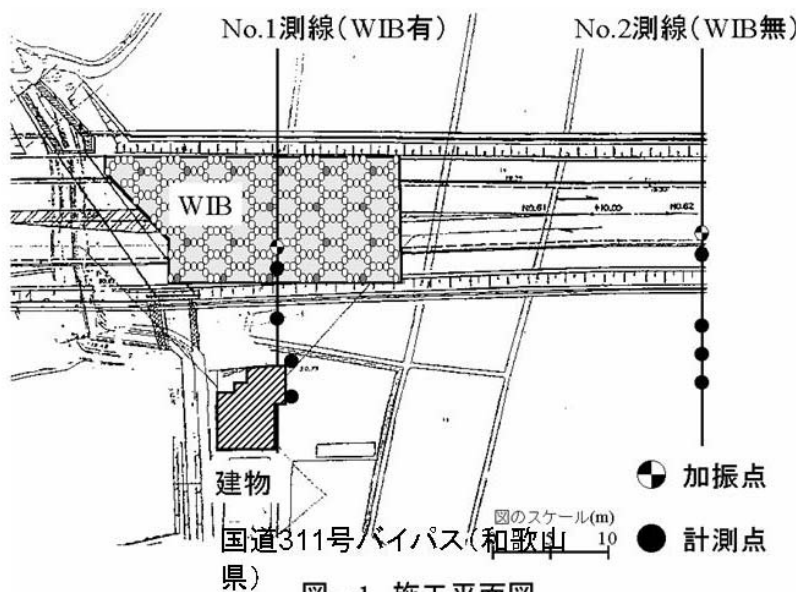
図-1 施工平面図
